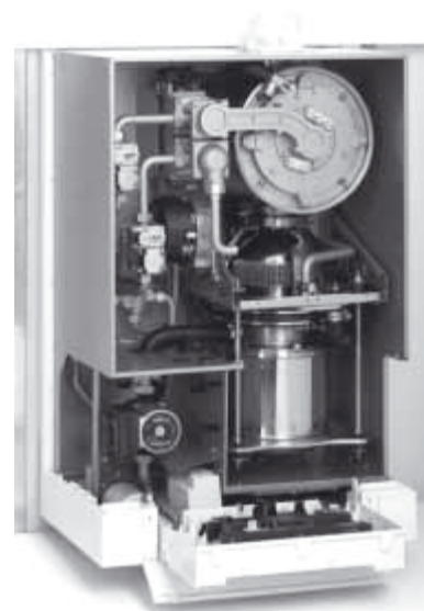
Stirlingův motor s plynovým kondenzačním kotlem
